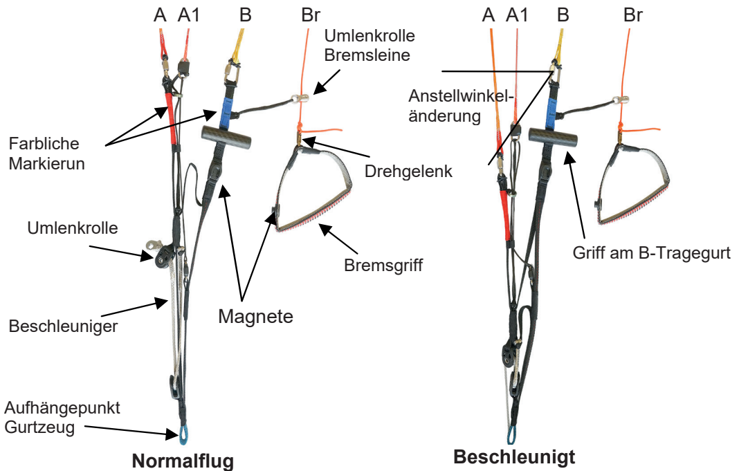
Tragegurte im Trimmflug und im beschleunigten Flug.
