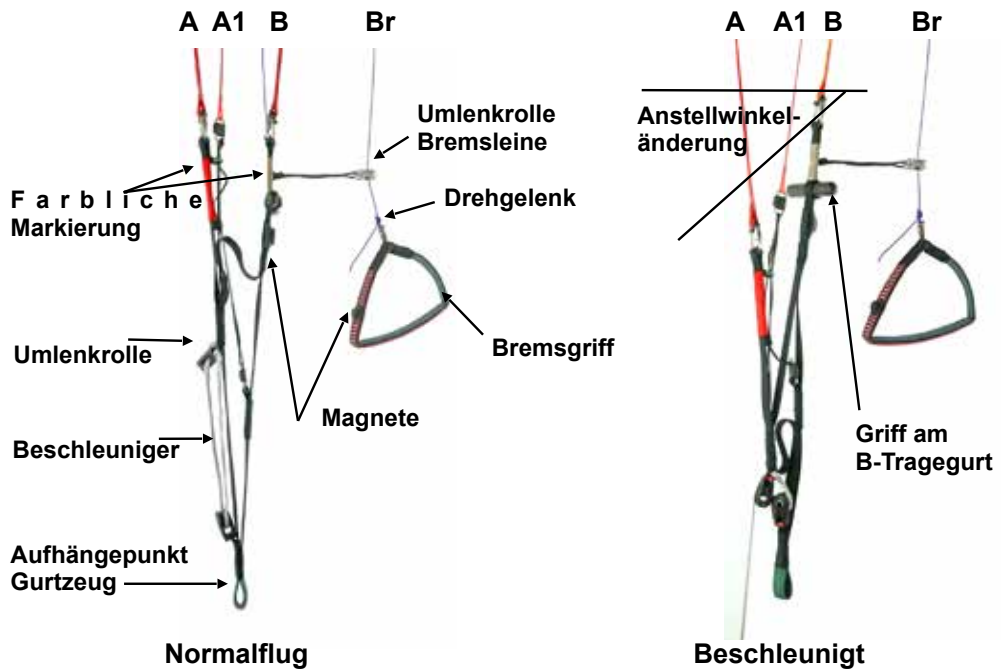
Tragegurte im Trimmflug und im beschleunigten Flug.
