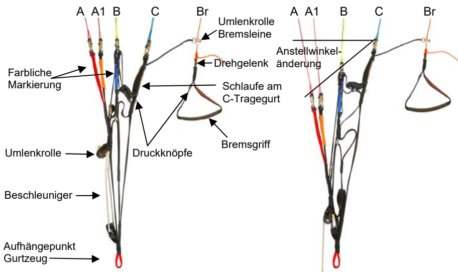
Normalflug
